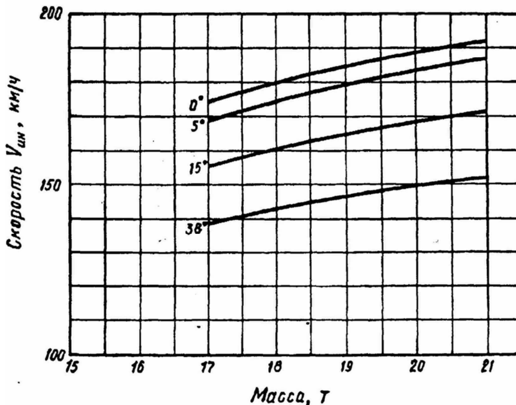
Рис. 5.7. Индикаторная скорость сваливания самолета Ан-24
