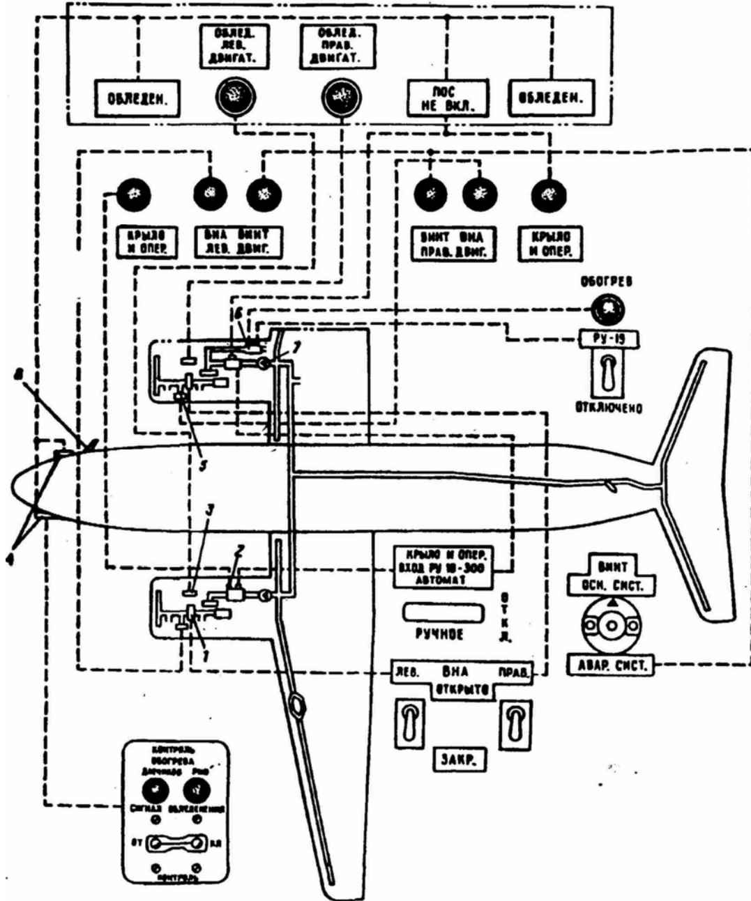
Рис 7.19. Принципиальная схема ПОС:
