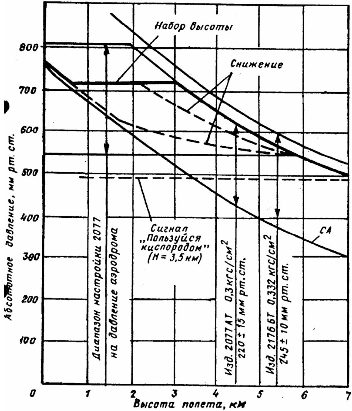
Рис. 7.17 График изменения давления в кабине.
