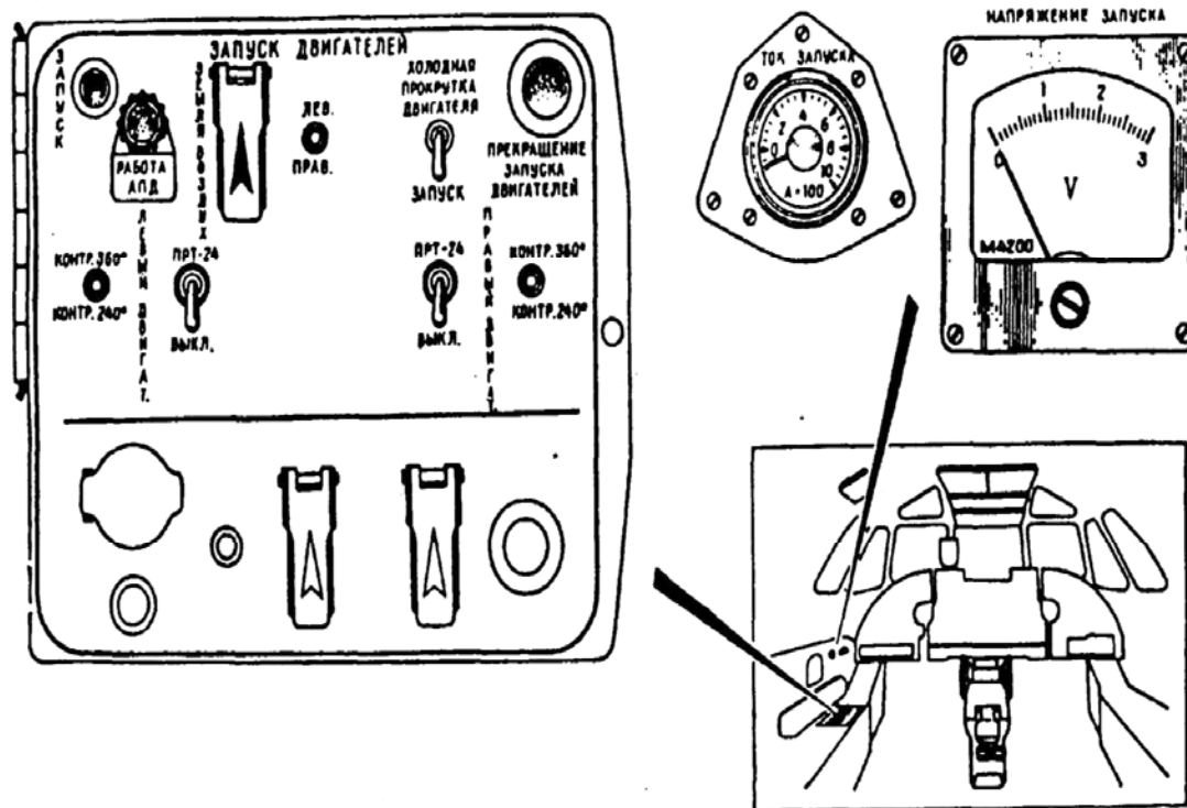
Рис. 7.1. Электрощиток управления запуска и приборы контроля запуска двигателей АИ-24
