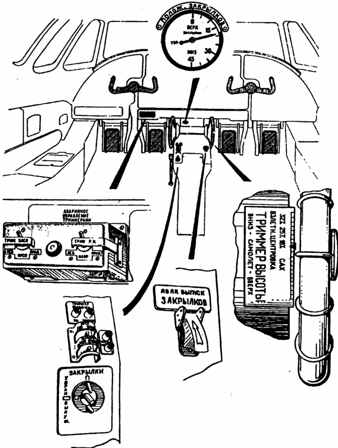
Рис. 7.14. Схема размещения органов управления
