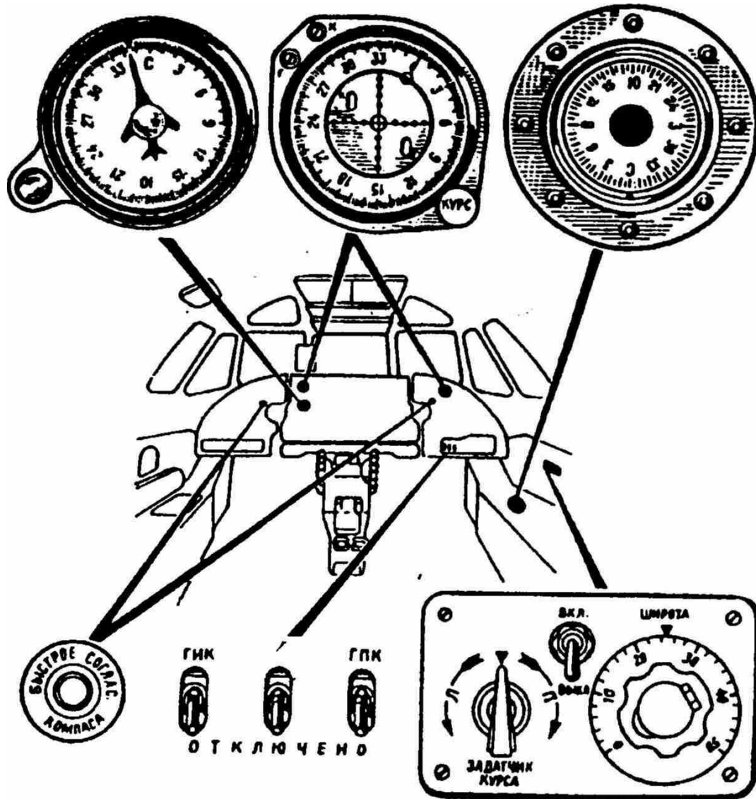
Рис. 7-30. Размещение органов управления и индикации курсовых приборов в кабине экипажа С этого момента указатель курса будет показывать ортодромический магнитный курс (ОМК) относительно меридиана аэродрома вылета.
