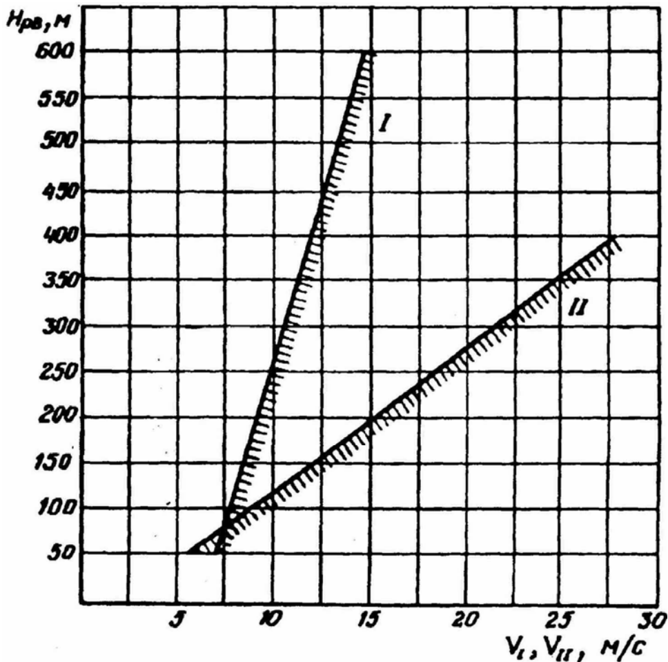
Рис. 7.34. Зоны включения сигнализации ССОС (I, II): H_{рв} — высота полета по радиовысотомеру; V_I — бароинерциальная скорость снижения; V_{II} — боарорadioинерциальная скорость снижения
