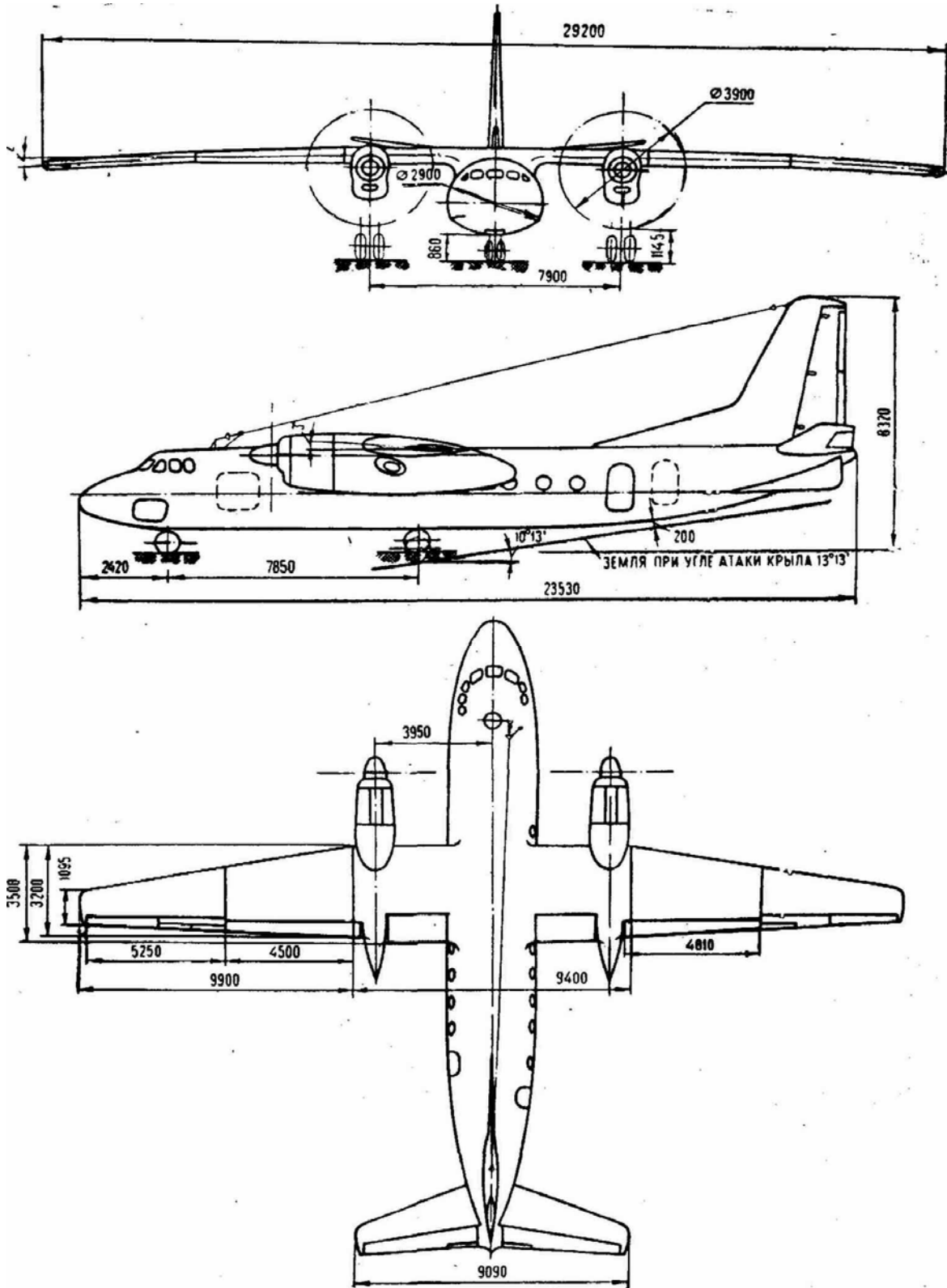
Рис. 1.1. Общий вид самолета
