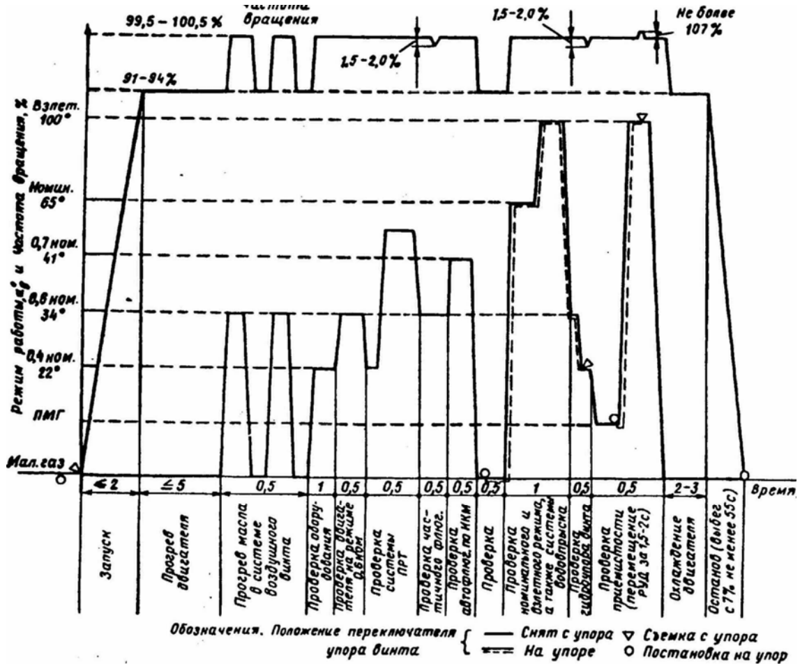
Рис. 7.3. График прогрева и опробования двигателей Ан-24 2-й серии (Ан-24Т)
